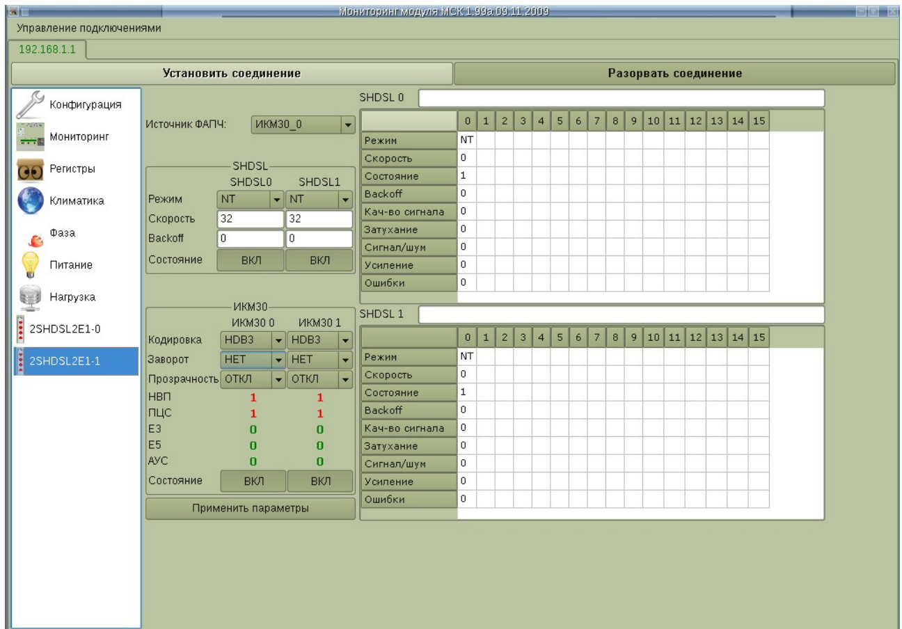
Рисунок 41: Окно 2SHDSL–2E1
