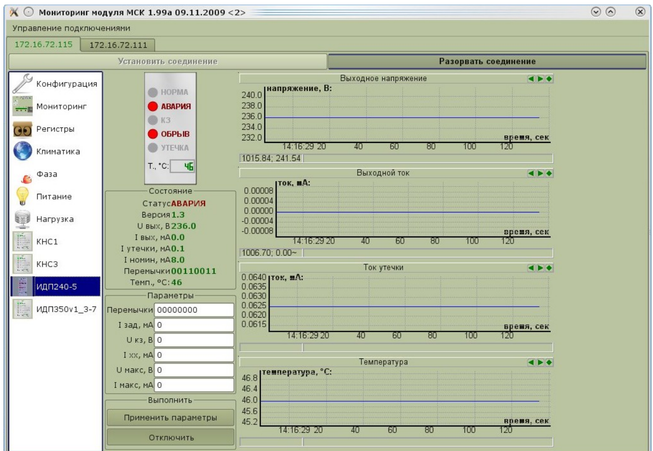
Рисунок 29: ИДП240
