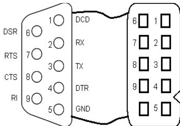
Рисунок 44: Переходник для МСК-БЭП
