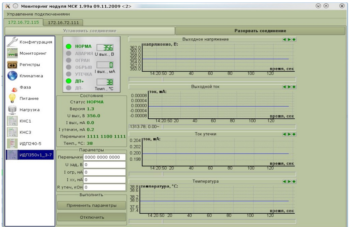
Рисунок 31: ИДП350v1.3
