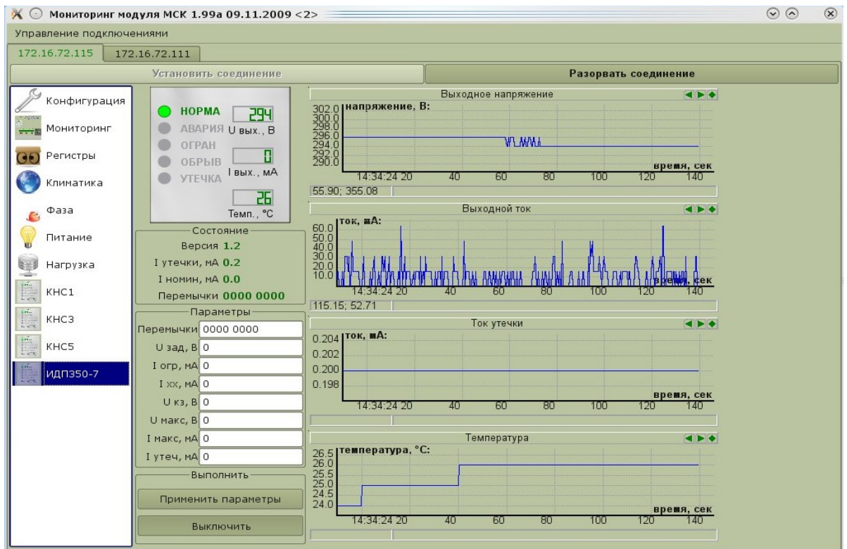
Рисунок 30: ИДП350
