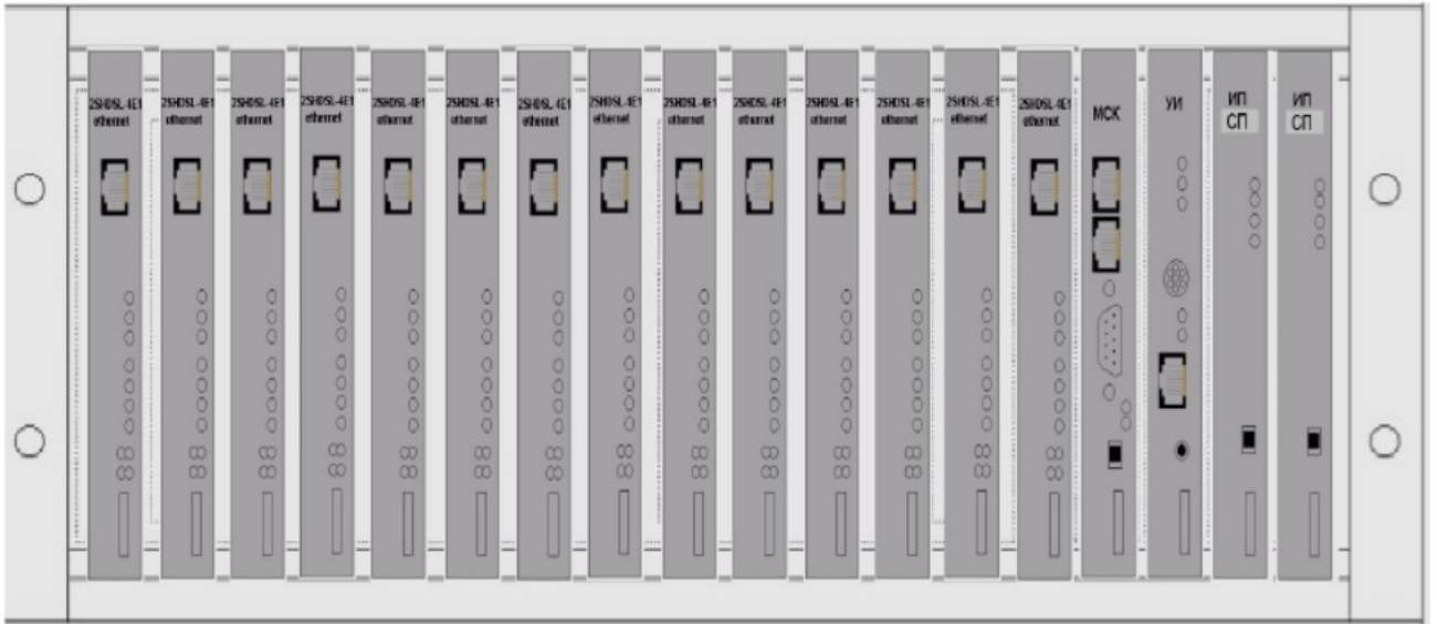
Рисунок 2: Блок УГМ-СП
