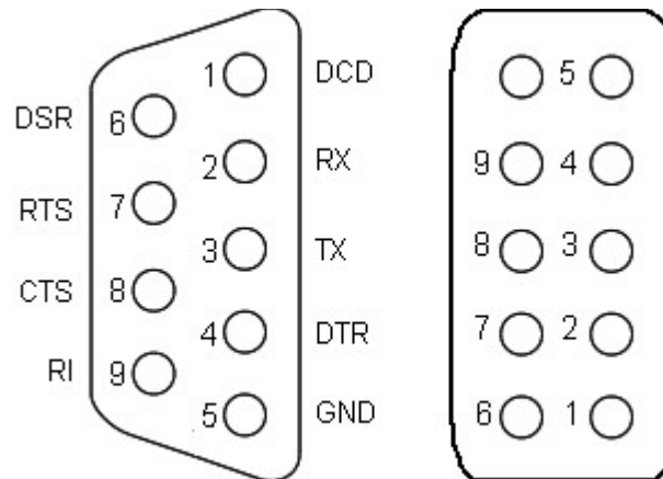
Рисунок 43: Разъемы RS-232 (COM)
