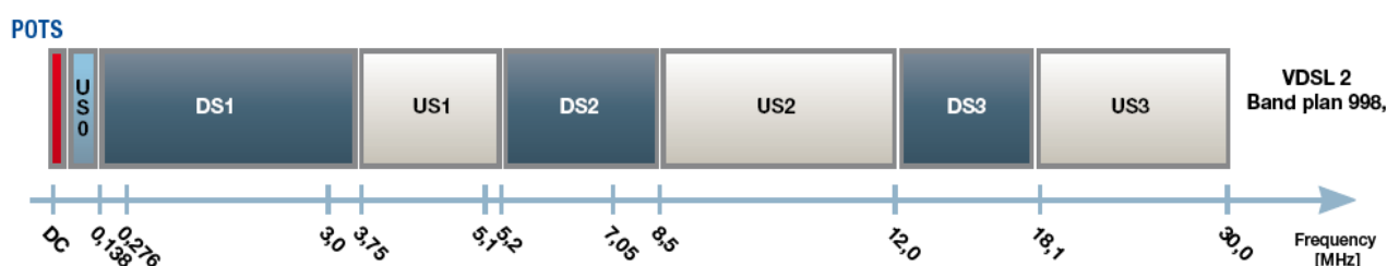
Рис. 1: Распределение частот VDSL2
